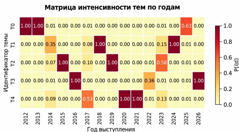
Рисунок 4. Матрица интенсивности
